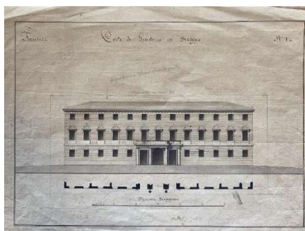
Progetto della facciata dell'ex Tribunale di Reggio Emilia dell'Arch. Domenico Marchelli (ASRE)
